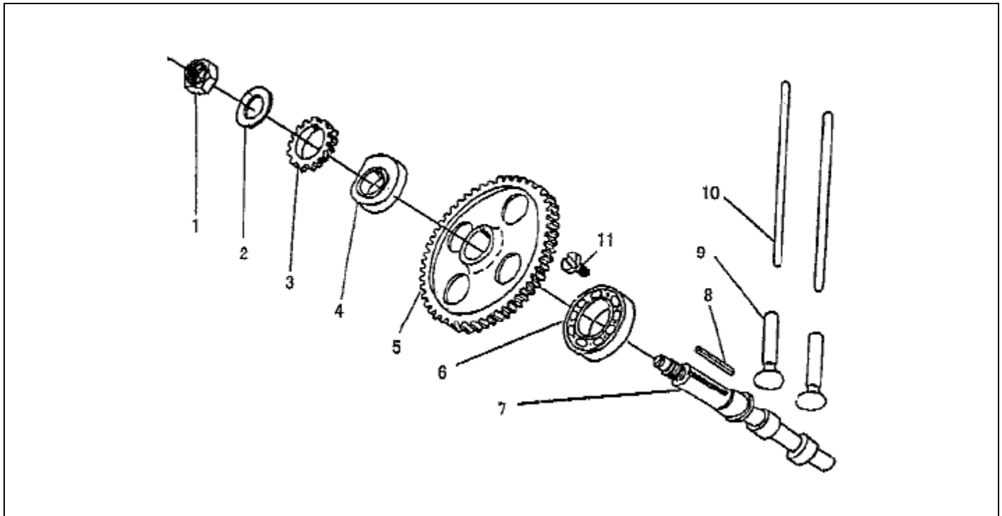
Fig. 6. Camshaft
